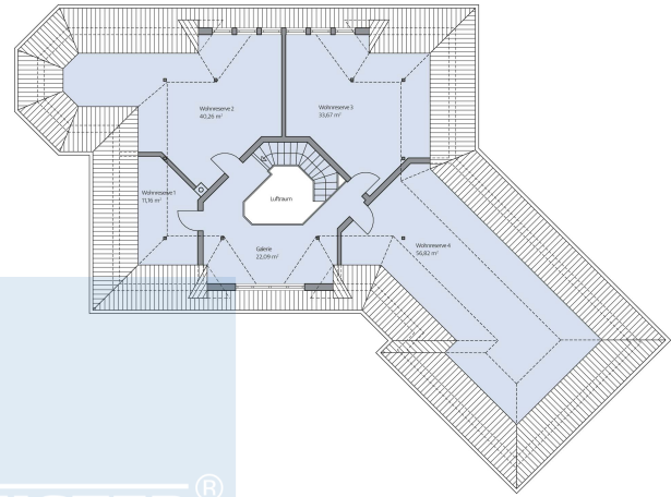
Haus Mühlberger Grundriss
