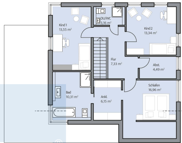
Haus Dietz Grundriss
