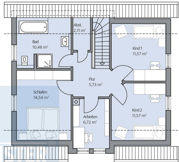
Haus Carl Grundriss
